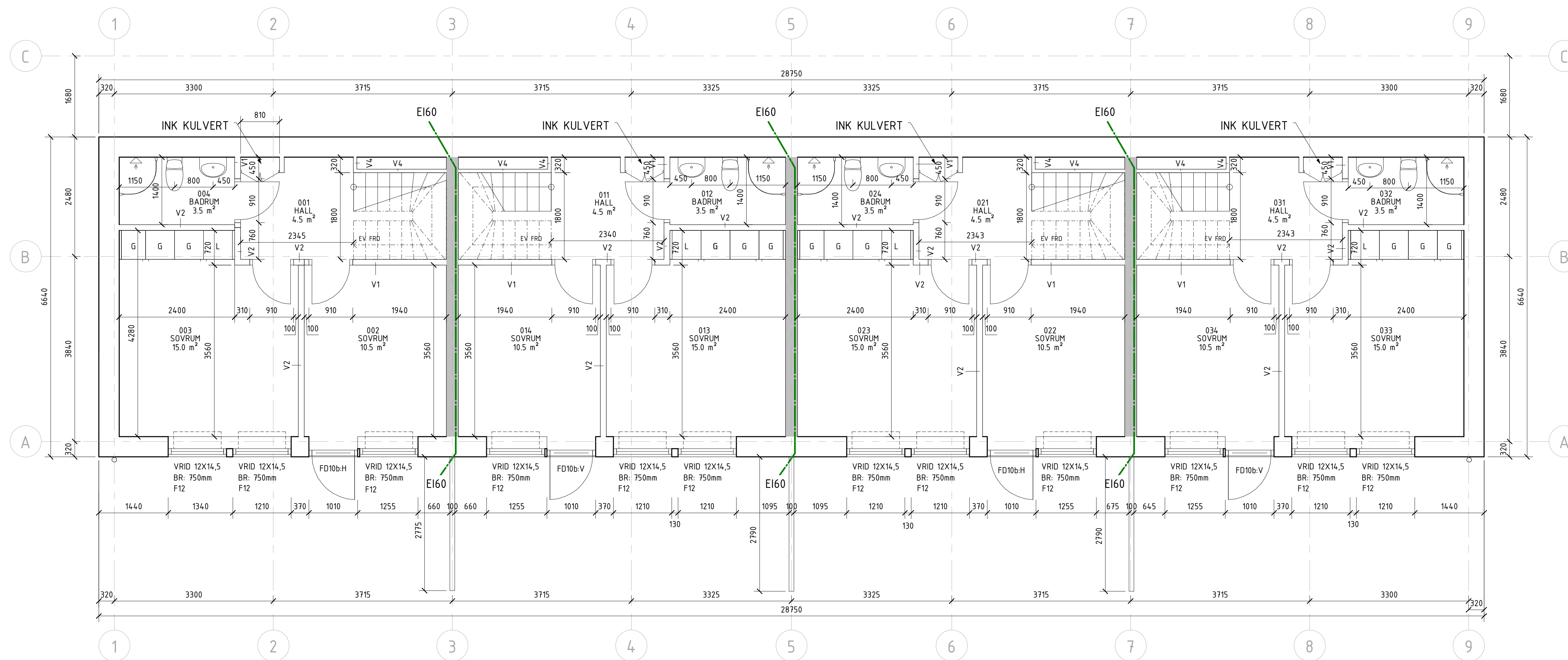
Plan 0 (Suterrängplan) SKALA 1 : 50
